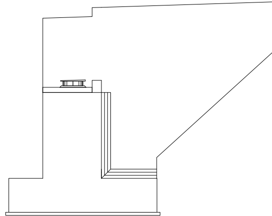
날개벽(우측)
