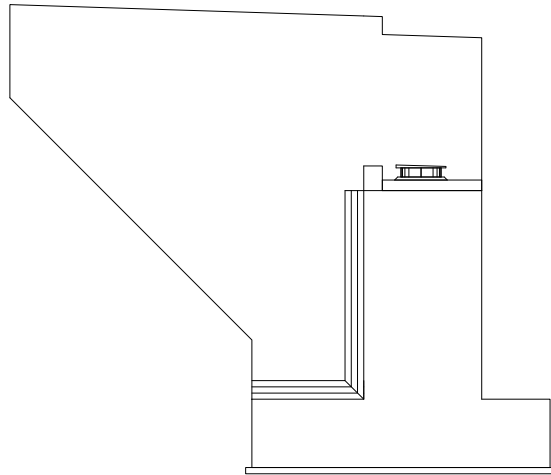
날개벽(좌측)
